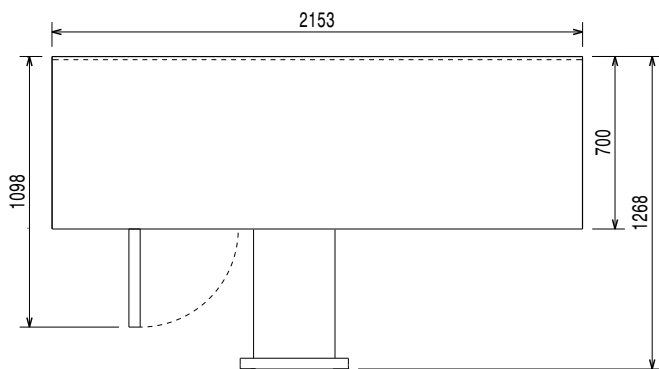
Felülnézet
